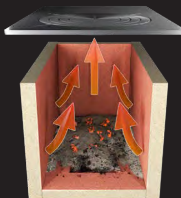
Phase 2: Restitution constante et progressive de la chaleur lorsque le feu est terminé
